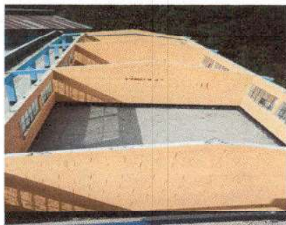
Foto 1: Sustrucción de Lámina, por lámina troquelada aluzinc calibre 26
